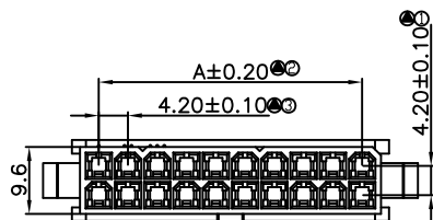
06~24Pin
