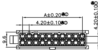
06~24Pin
