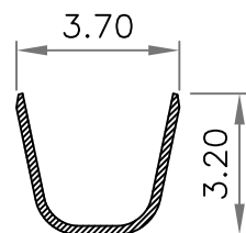
A-A Section
