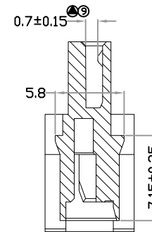
SEC:A-A
