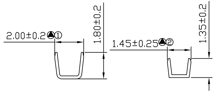
A-A SECTION
