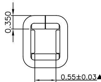
SEC:D-D SC 3:1
