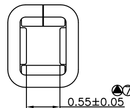
SEC:D-D SC 3:1
